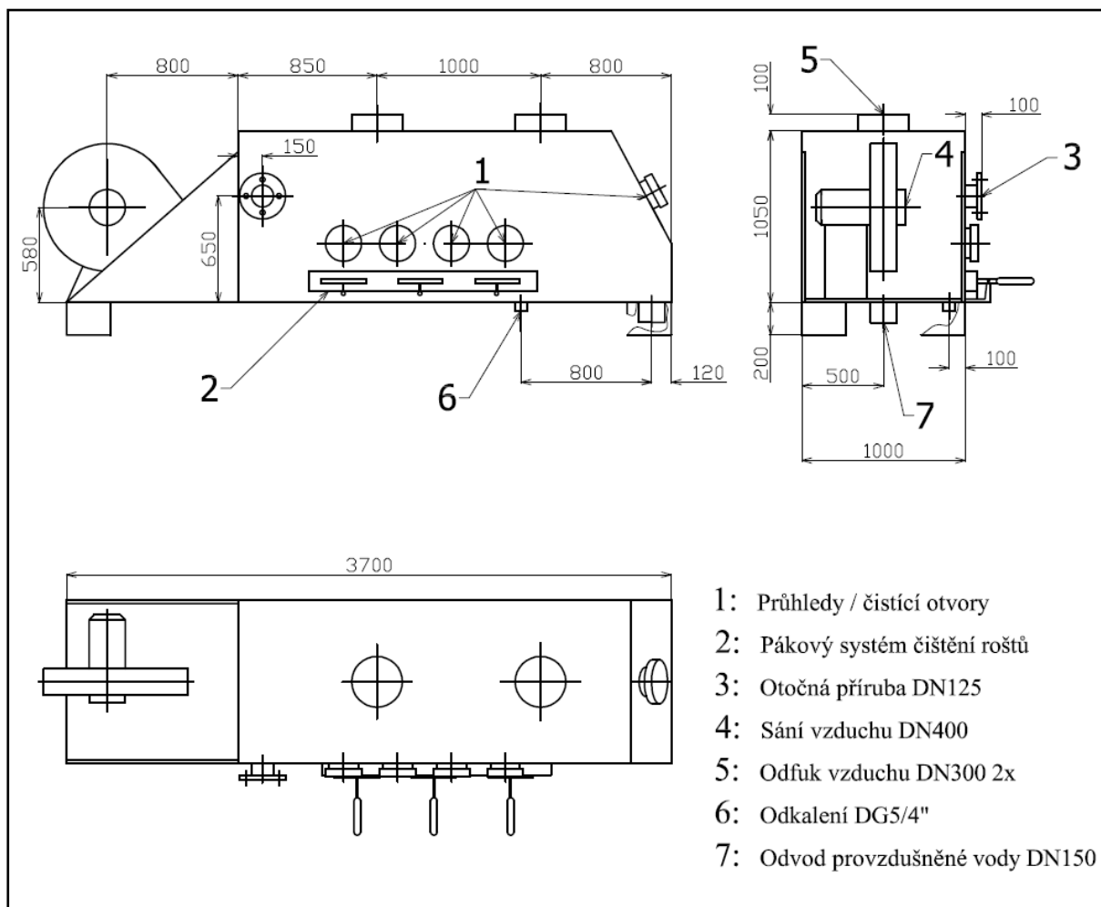
Obr. č2: Zástavbové rozměry Bubla 9V
