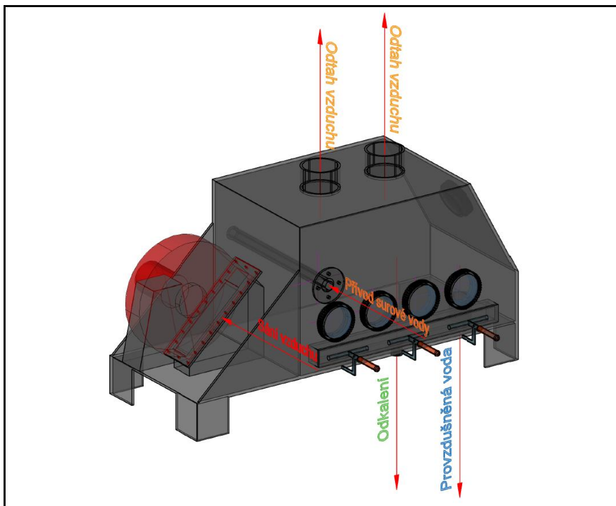
Obr. č1: Schéma zapojení aerátoru typu Bubla
